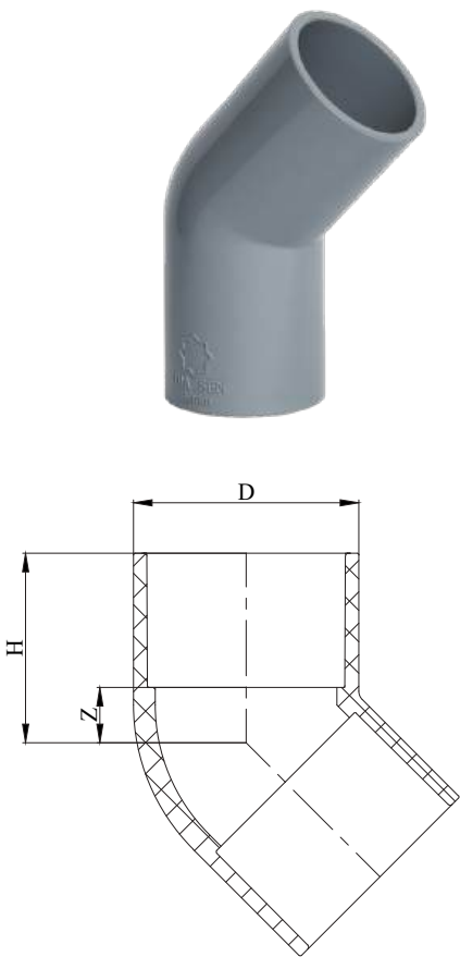
LỖI 45°Elbow
